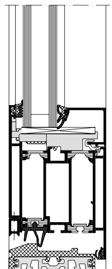
Horizontale doorsnede Schüco Deur ADS 75 SimplySmart Coupe horizontale porte Schüco ADS 75 SimplySmart
